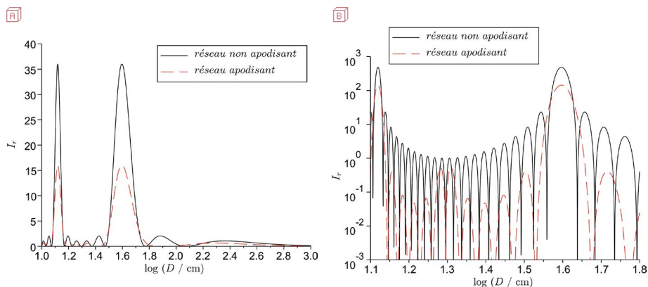
Figures 12A et 12B - Comparaison des intensités relatives données par un réseau apodisant (pointillé rouge) et par un réseau non apodisant (trait plein noir) dans les cas N=3 ( Q=2 ) et N=11 ( Q=6 ). Pour plus de lisibilité, l'échelle en ordonnées de la figure 12B est logarithmique.
