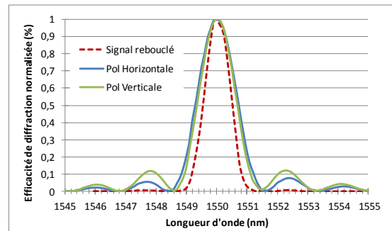
Fig. 4 : Efficacités de diffraction normalisées en fonction de la longueur d'onde pour les trois configurations expérimentales.
