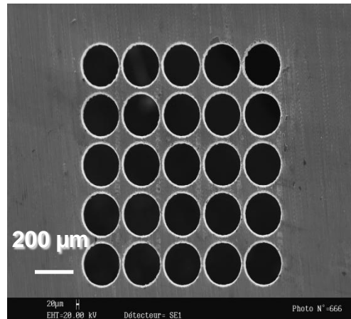
Inox Trous 200 µm épaisseur 100 µm
