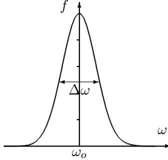
Figure 9 - Profil gaussien
