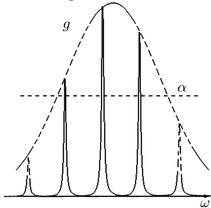
Figure 10 - Modes longitudinaux
