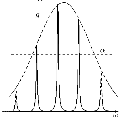
Figure 10 - Modes longitudinaux
